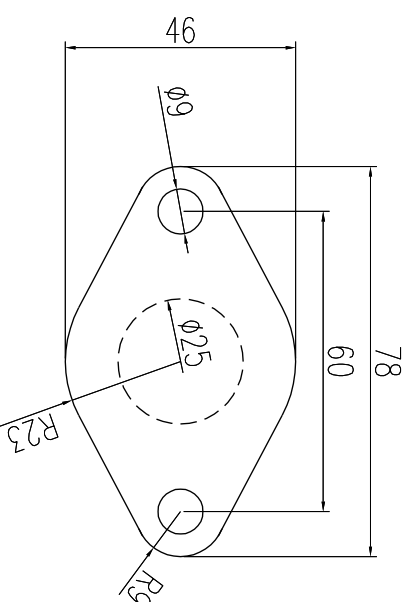
OSA 2 EGR pakosarjan laippa
